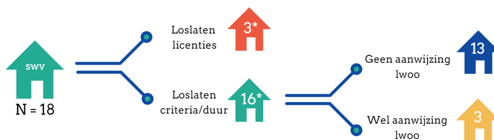
Figuur 3-1 Varianten van opting out
